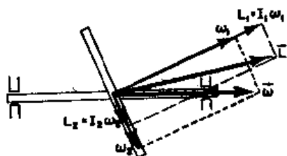
图 20-6 一个转动物体的角动量并不一定平行于角速度
