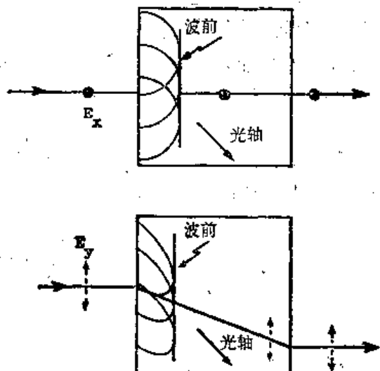
图 33-7 上图表示通过双折射晶体的寻常光线路径,非常光线路径画于下图中. 光轴位于纸面上
