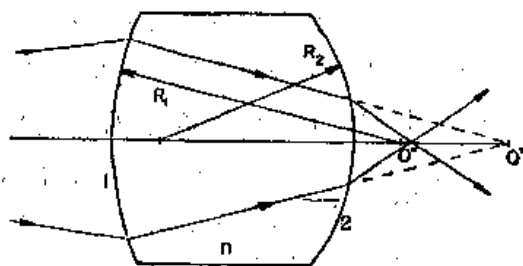
图 27-5 双面透镜成像
