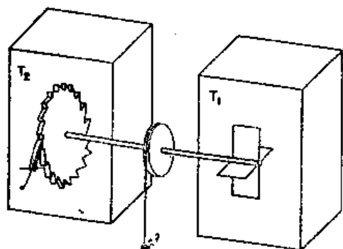
图 46-1 棘轮和掣爪
