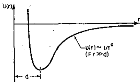
图 14-3 两个原子之间的势能与它们之间的距离的关系
