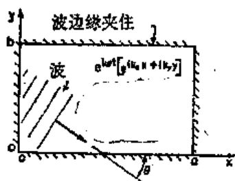
图 49-4 振动的矩形板
