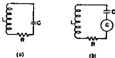
图 41-2 高 Q 值谐振电路
