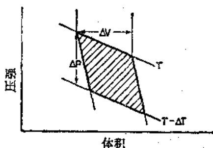
图 45-1 卡诺循环的压强-体积图. 标有 T 和 T-\Delta T 的曲线是等温线; 较陡的曲线是绝热线. \Delta V 是在恒定温度 T 下加入到气体中的 \Delta Q 的热量所引起的体积改变. \Delta P 是在恒定体积下温度从 T 变为 T-\Delta T 所引起的压强改变
