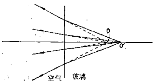
图 27-4 一平表面把发自 O' 的光重新成像为 O
