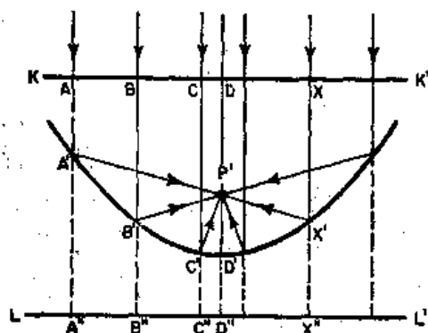
图 26-12 抛物面镜
