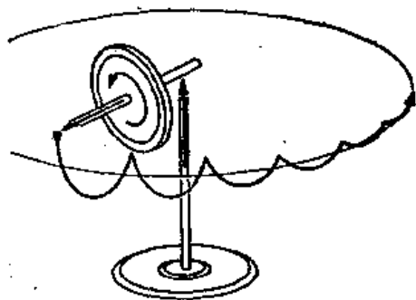
图 20-5 原来被紧紧抓住的回转器刚放开之后, 在重力的作用下, 其轴端的实际运动情况
