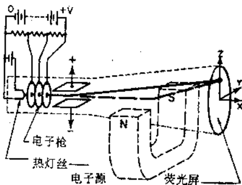
图 12-3 电子束管
