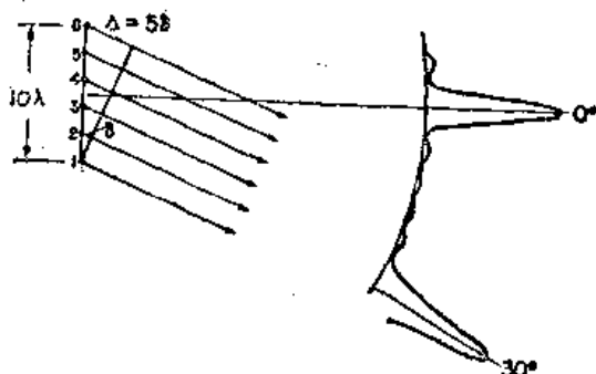
图 29-8 六个偶极子天线装置和它的强度分布图的一部分
