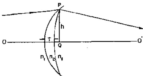
图27-6 两个曲率半径都为正的薄透镜
