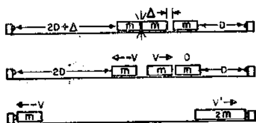
图 10-6 验证以速度 v 运动的质量为 m 的物体与一个质量相同的静止物体碰撞后结合在一起以质量 2m 、速度 \frac{1}{2}v 运动的实验
