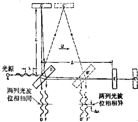
图 15-2 迈克耳孙-莫雷实验的示意图
