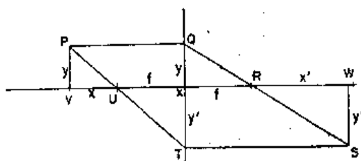
图 27-7 薄透镜成象的几何图
