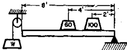
图 4-6 一端支撑着的荷重杆
