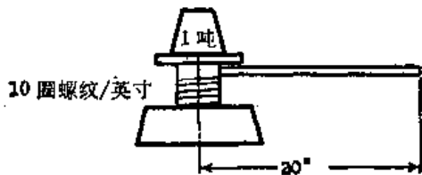
图 4-5 螺旋起重器
