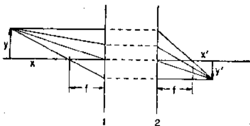
图 27-8 光学系统主平面示意图
