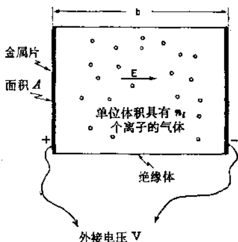
图 43-2 电离气体的电流
