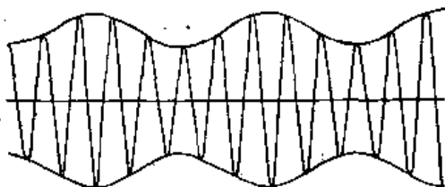
图 48-4 调制载波。在此简图中, \frac{\omega_c}{\omega_m} = 5 。 在实际的无线电波中, \frac{\omega_c}{\omega_m} \sim 100
