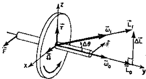
图 20-2 回转器
