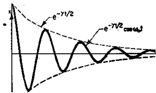
图 24-1 一个阻尼余弦振动
