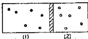
图 39-2 两种不同的单原子气体的原子被一可移动的活塞隔开
