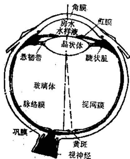
图 35-1 眼睛
