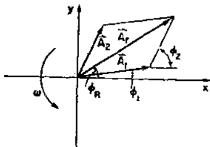
图29-9 合成两个余弦波的几何方法。 想象整个图以角频率 \omega 逆时针旋转着
