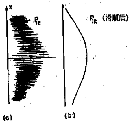
图 37-5 子弹的干涉实验
