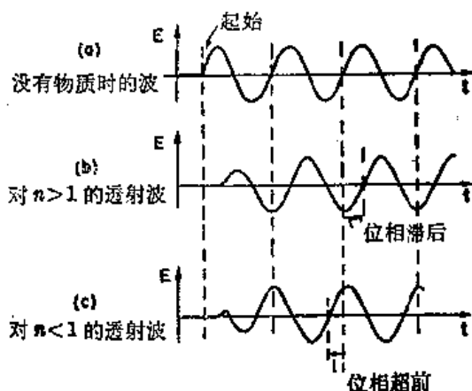
图 31-4 波“信号”
