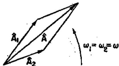
图 48-2 两个相同频率复矢量的合成
