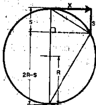
图 7-4 指向圆形轨道中心的加速运动。根据平面几何, x/s = (2R-s)/s = 2R/s , 其中 R 是地球的半径 (4000 英里), s 是每秒“水平通过”的距离, s 是每秒“下落”的距离 (16 英尺)
