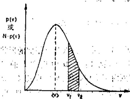
图 6-9 气体中分子的速度分布
