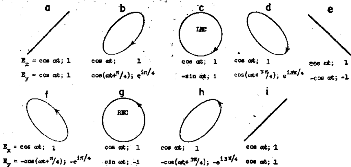
图 33-2 等振幅而相对位相不同的 x 振动与 y 振动的迭加. E_x 与 E_y 两个分量用实数与复数两种符号表示
