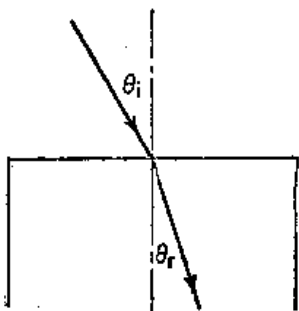
图 26-2 当光从一种介质进入另一种介质时发生的折射
