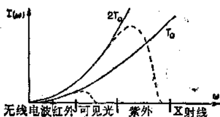
图 41-4 在两种温度下,黑体辐射的强度分布。实线表示按照经典物理所给出的分布,虚线表示实际的分布
