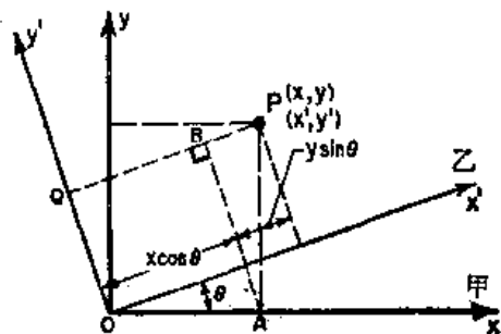
图 11-2 角方位不同的两个坐标系
