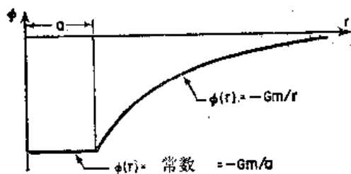
图 14-4 由半径为 a 的球壳所引起的势能
