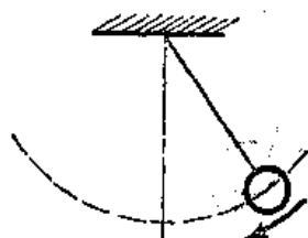
图 4-7 单摆
