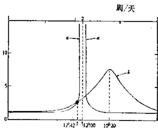
图 23-6 大气层对外来激发的响应。如果大气层 S_2 -潮汐是由万有引力引起的, a 就是这种条件下所需的响应; 峰值的放大率是 100:1, b 是从 2S_2 -潮汐观察的倍数和位相导出的
