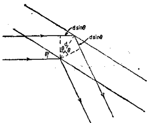
图 38-4 晶面对波的衍射
