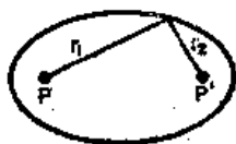
图 26-11 椭圆面镜
