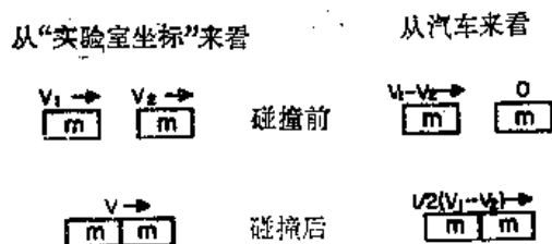
图 10-5 质量相等的物体进行的另一种非弹性碰撞的两种情况
