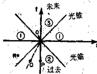
图 17-3 在原点周围的空时区域
