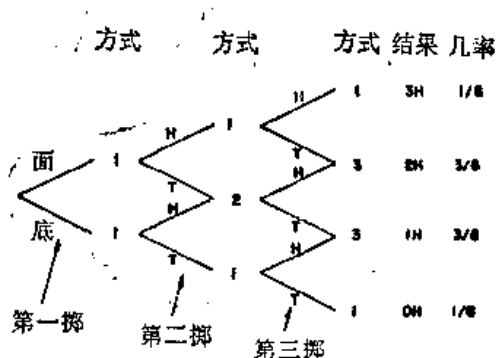
图 6-3 在抛掷三次的游戏中,能得到 0, 1, 2, 3 次正面的方式数目的图解表示
