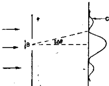
图 38-2 粒子穿过狭缝的衍射
