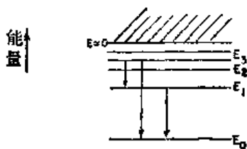
图38-9 原子的能级图(表示 n 种可能的跃迁)
