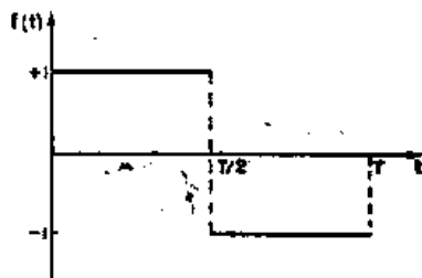
图 50-3 方波函数
