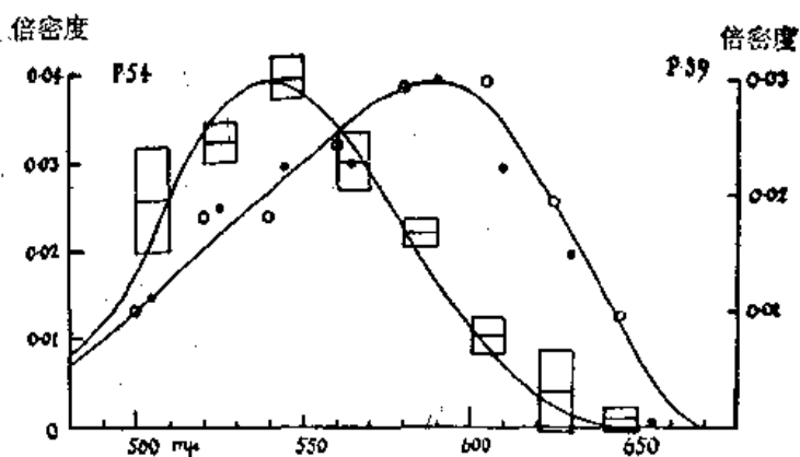
图 35-10 患红色盲的人的眼睛(方块)和正常眼睛(点)的色素吸收光谱
