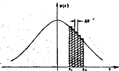
图 6-8 无规行走中所通过的距离 D , 它位于 x_1 与 x_2 之间的几率就是曲线 p(x) 下方从 x_1 到 x_2 的面积
