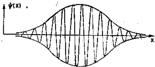
图48-6 定域波列
