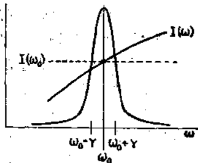
图 41-3 式 (41.10) 被积函数的图式. 图中的峰为谐振曲线 1/[(\omega - \omega_0)^2 + \gamma^2/4] . 作为一个很好的近似, I(\omega) 可用 I(\omega_0) 来代替
