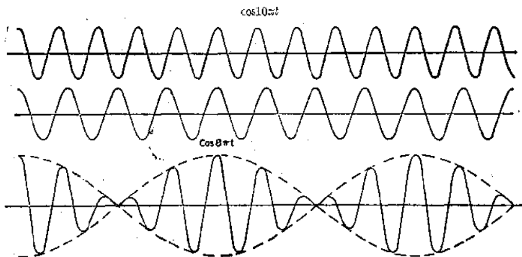
图 48-1 频率比为 8:10 的两列余弦波的迭加。图中各个“拍”内的图样精确重复这一点在一般情况下并不具有代表性
