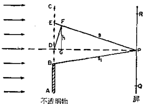
图 30-7 远处光源将一不透明物的影子投射于屏上
