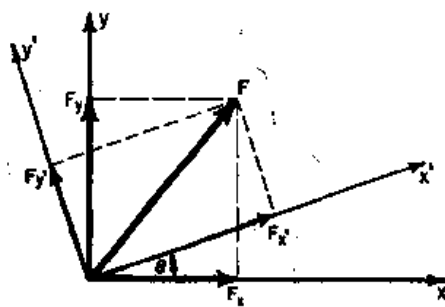
图 11-3 在两个坐标系中力的分量
