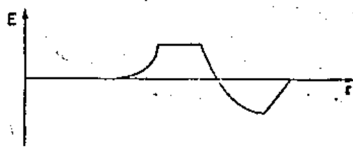
图 29-3 下一时刻的电场与位置的关系(忽略 1/r 引起的改变)
