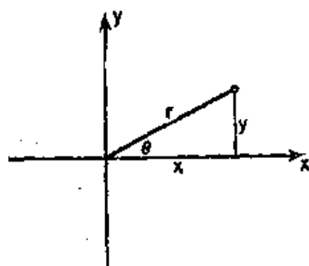
图 22-2 x + iy = re^{i\theta}
