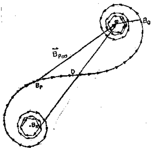
图 30-8 位相延迟与离上图 D 点的距离平方成正比的许多同相振子振幅的迭加
