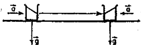
图 12-4 赝力的实例
