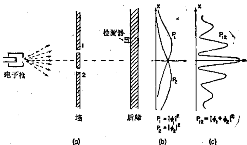
图 37-3 电子的干涉实验
