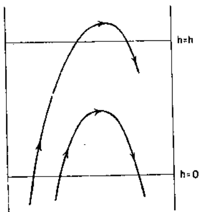
图 40-4 只有那些具有足够速度的分子从 h=0 向上移动才能够到达 h 的高度
