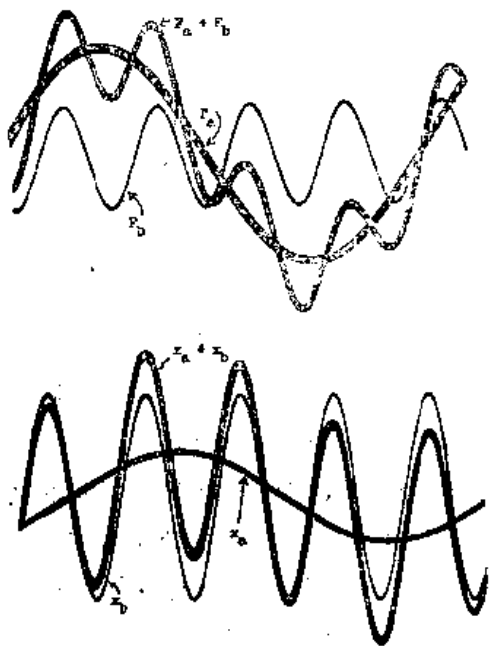
图 25-1 线性系统迭加原理的一个例子
