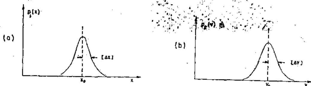
图 6-10 观察一个粒子的位置与速度时的几率密度
