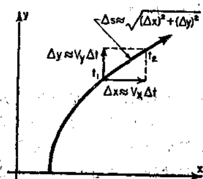
图 8-3 物体二维运动的描述和它的速度的计算
