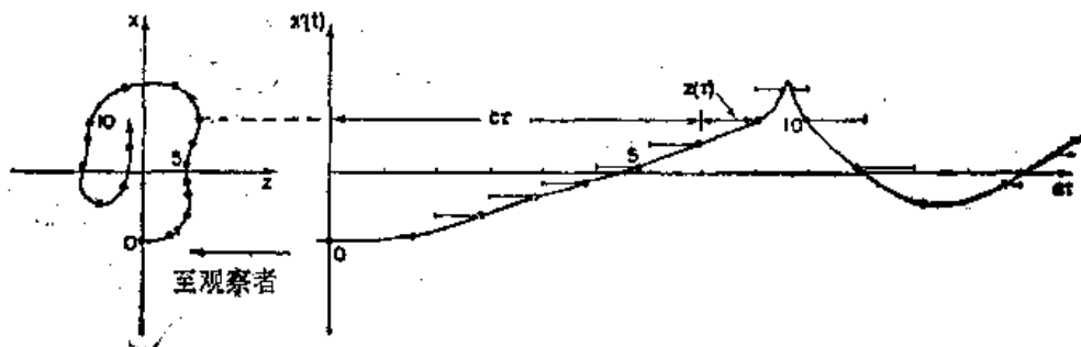
图 34-2 由方程 (34.5) 求 x'(t) 的几何解法
