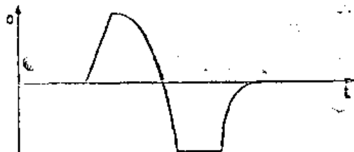
图 29-2 某电荷的加速度与时间的关系
