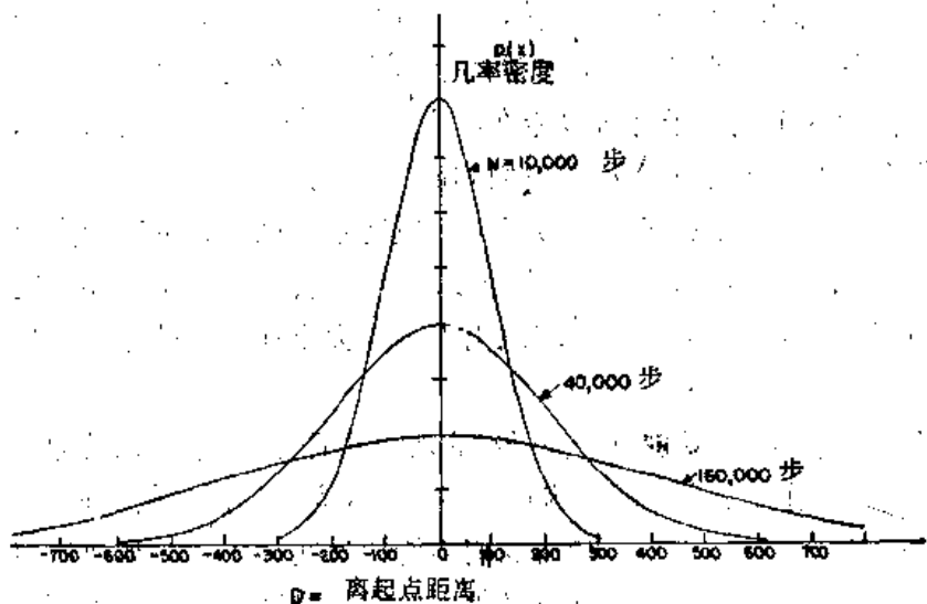
图 6-7 在步数为 N 的无规行走中停止在从起点算起的距离 D 处的几率密度 ( D 是用方均根步长为单位来量度的)
