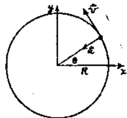
圖 21-2 以恒速在一圓形軌道上運動的粒子
