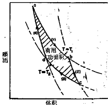
图 44-6 卡诺循环
