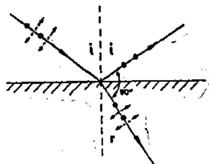
图 33-4 在布儒斯特角下线偏振光的反射。虚线箭头表示偏振方向;圆点表示偏振垂直纸面
