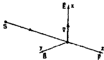
图 34-13 作用在受电场驱动 的电荷上的磁力沿着光束方向
