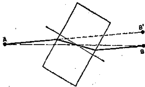
图 26-6 当一束光通过一块透明板时, 它被偏移了
