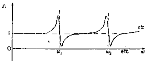
图 31-5 折射率与频率的关系
