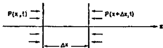
图 47-4 作用在垂直于 x 的单位面积上的压强在正 x 方向上所产生的净力是 -\left( \frac{\partial P}{\partial x} \right) \Delta x
