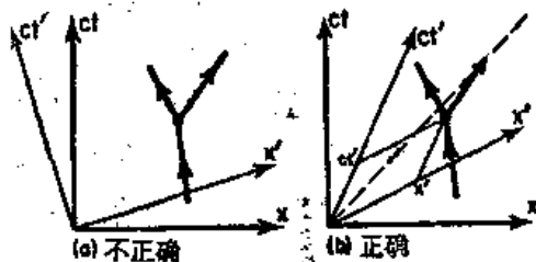
图 17-2 对一个蜕变粒子的两种看法
