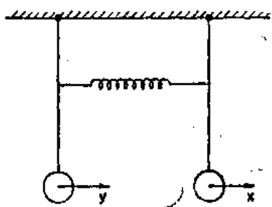
图 49-5 两个耦合摆
