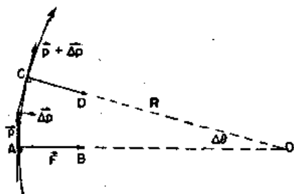
图 34-4 带电粒子在均匀磁场中沿圆周(或螺旋线)运动
