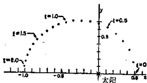
图 9-6 由计算所得的行星绕日运动
