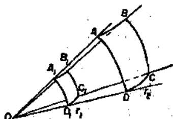
图 29-4 包含在角锥 OABCD 中的能流与测量的距离 r 无关
