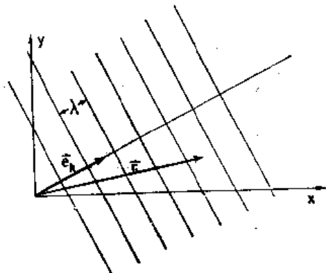
图 34-11 沿倾斜方向传播的平面波
