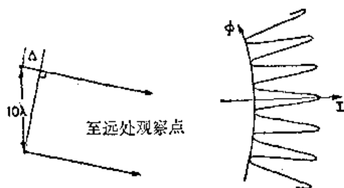
图 29-7 两个相距 10\lambda 的偶极子 (a) 强度分布图
