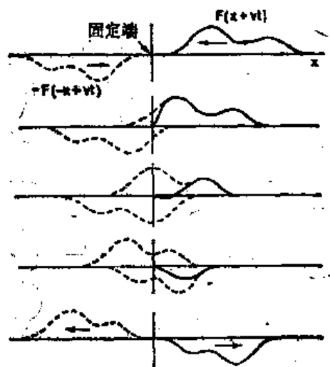
图 49-1 把波的反射看作为 两个行波的迭加
