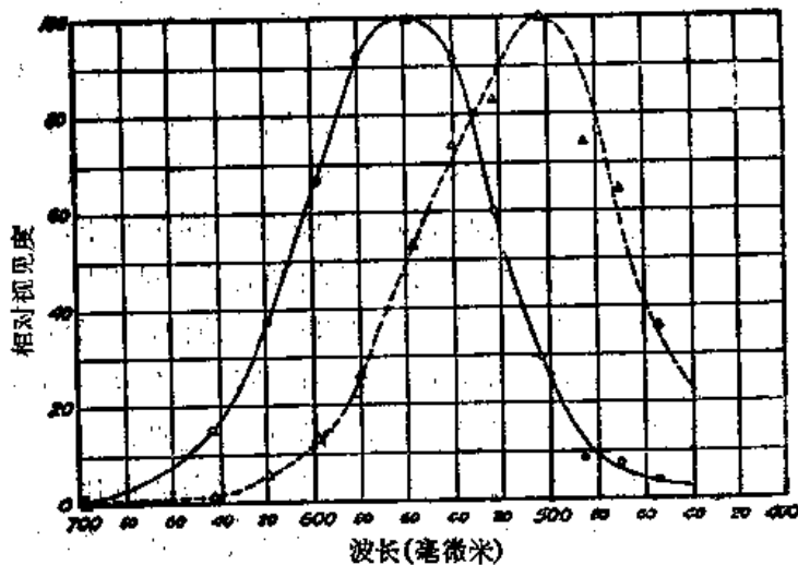
图 35-3 眼睛的光谱灵敏度。虚线——杆状细胞;实线——圆锥细胞
