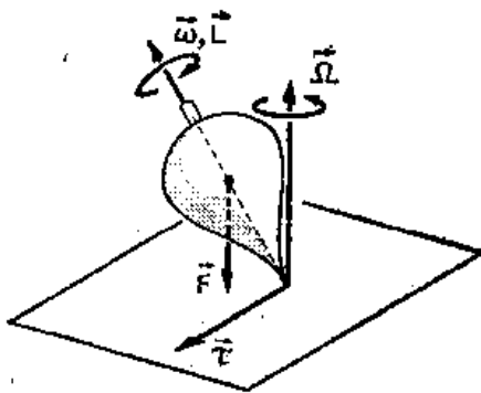
图 20-3 一个快速旋转的陀螺 注意: 转矩矢量的方向就是进动的方向
