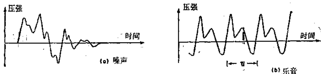
图 50-1 压力与时间的关系。(a) 噪声; (b) 乐音
