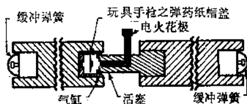
图 10-2 带有爆破作用气缸附件的滑块截面图
