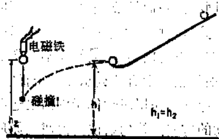
图 7-3 演示垂直与水平运动互不相关的仪器装置
