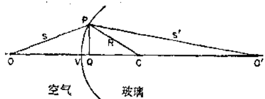
图 27-2 单折射面聚焦
