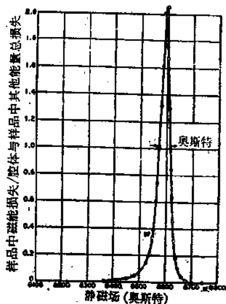
图 23-8 在顺磁有机化合物中，磁能损失与外加磁场强度的关系
