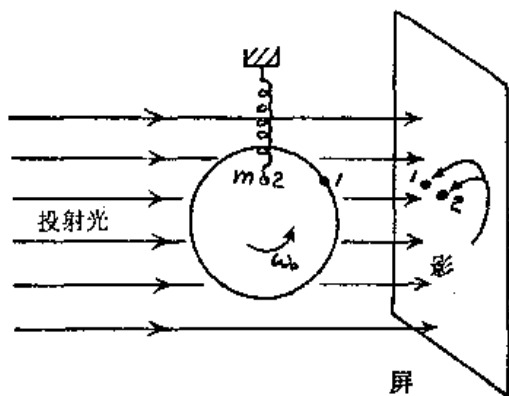
圖 21-3 演示簡諧運動和勻速圓周運動之間等同性的實驗
