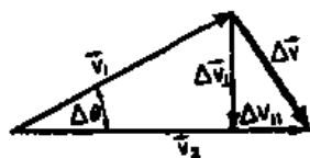
图 11-8 计算加速度的矢量图
