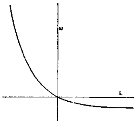
图46-2 棘轮的角速度与力矩的关系
