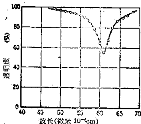
图 23-7 通过一个薄氯化钠膜 ( 0.17\mu\text{m} ) 的红外辐射透射
