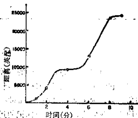
图 8-1 汽车的距离-时间曲线
