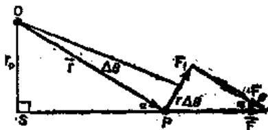
图18-2 一个力产生的转矩
