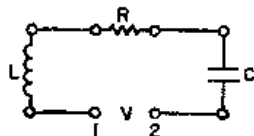
图 23-5 由电阻、电容和电感组成的振荡电路
