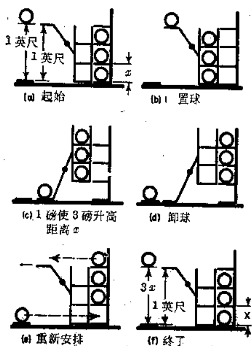
图 4-2 一种可逆机
