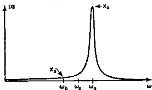
图 25-3 尖锐的谐曲线
