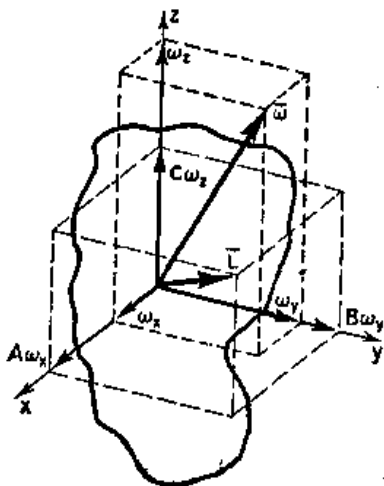
图 20-7 一个刚体的角速度和角动量 ( A > B > C )
