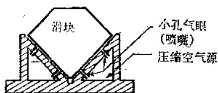
图 10-1 线性气垫侧视图
