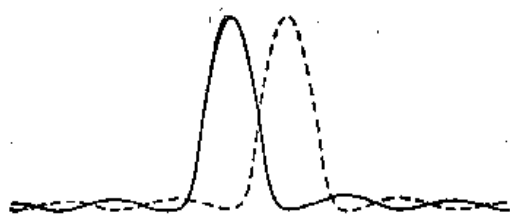
图 30-6 瑞利判据的说明.一个花样的极大值落在另一个花样的第一极小值上
