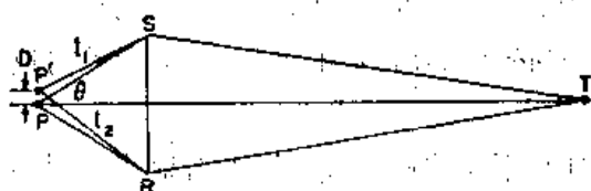
图 27-9 光学系统的分辨本领
