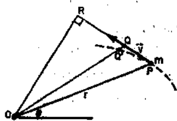
图 18-3 一个围绕轴 O 运动的质点
