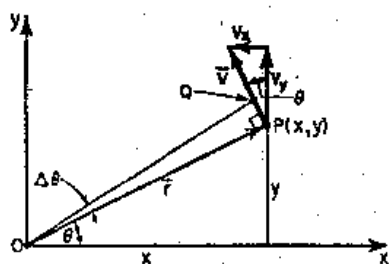
图 18-1 二维转动动力学图示
