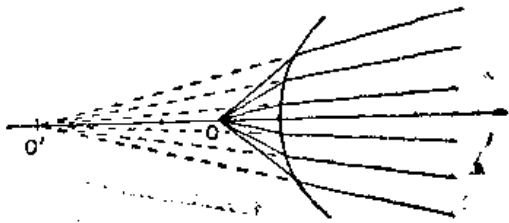
图 27-3 虚象
