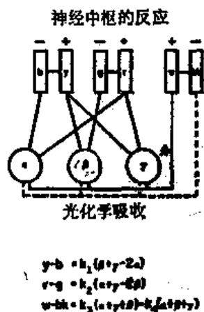
图 36-2 根据色视觉“反色”理论的神经连结
