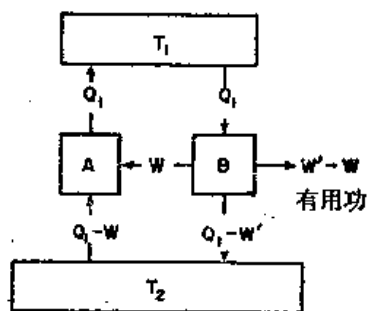
图44-7 热机 B 使可逆机 A 反向运转
