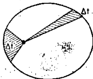
图 7-2 开普勒的面积定律
