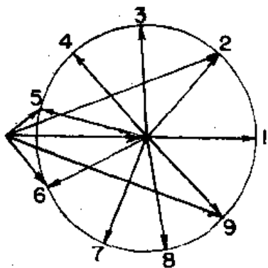
图 48-3 以一个旋转矢量为参考系来看, 两个不同频率的复矢量的合成。图中绘出了缓慢旋转的矢量的九个相继位置
