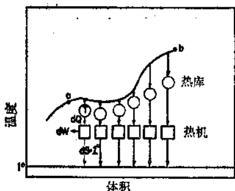
图 44-10 在可逆变化中熵的改变
