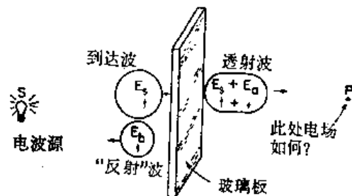
图 31-1 通过一层透明物质的电波
