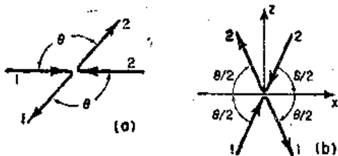
图 16-2 两个以相等速率、相向运动的相同粒子所发生的弹性碰撞的两种方式
