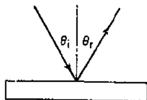
图 26-1 入射角等于反射角
