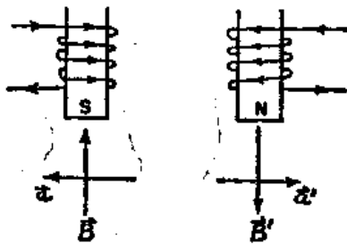
图 52-4 磁铁与其镜像
