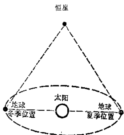
图 5-5 利用地球轨道的直径作为基线,可以用三角法测量靠近地球的恒星的距离
