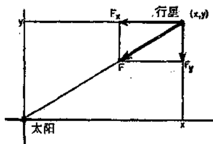
图 9-5 作用在行星上的太阳引力
