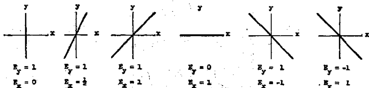
图 33-1 同位相的 x 振动与 y 振动的合成
