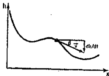
图 13-1 物体在重力作用下在一 无摩擦的曲线上的运动
