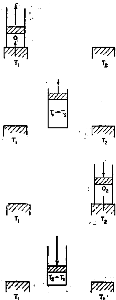
图 44-5 卡诺循环中的各个步骤
