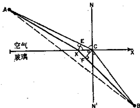
图 26-4 费马原理对折射的说明
