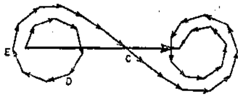
图 26-14 许多邻近路径的几率振幅总和
