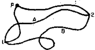
图 14-2 力场中二点之间的可能途径
