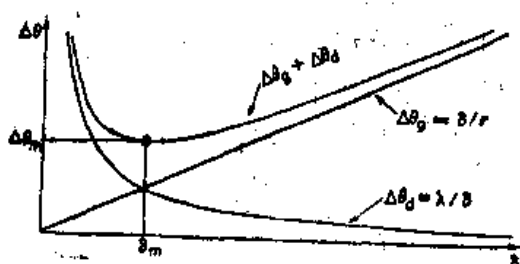
图 36-9 小眼的最佳大小为 \delta_m
