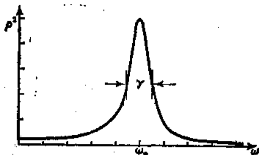
图 23-2 \rho^2 对于 \omega 的关系图
