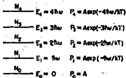
图 41-5 谐振子的能级是等间距的:
