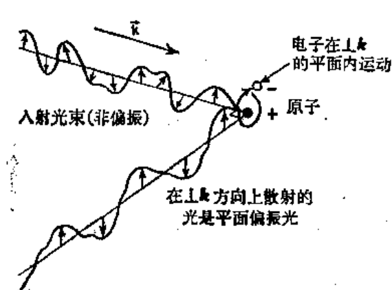
图 32-3 说明垂直于入射光束方向上散射的光的偏振化起因的图
