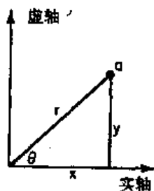
图 23-1 一个复数可以用“复平面”上的一个点来表示
