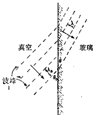
图 31-2 折射与速度改变之间的关系
