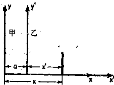
图 11-1 两个平行坐标系
