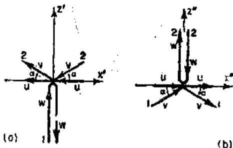
图 16-3 从运动汽车上看上去的碰撞时另外两种方式
