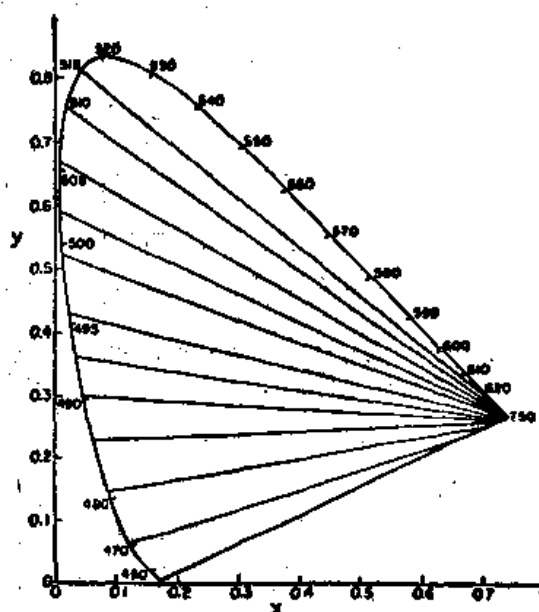
图 35-7 被患红色盲的人搞混乱的颜色轨迹
