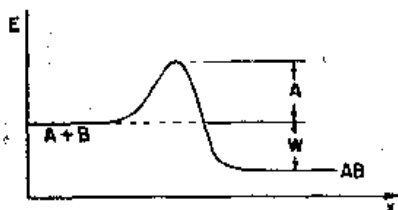
图 42-1 化学反应 A+B \rightarrow AB 的能量关系
