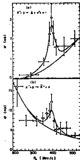
图 23-11 动量与反应截面的依赖关系。 (a) K^- + p \rightarrow \Lambda + \pi^+ + \pi^- 和 (b) K^- + p \rightarrow K^0 + n 。在 (a) 和 (b) 中下面的曲线代表假定的非共振背景,而上面的曲线是在背景上再加共振
