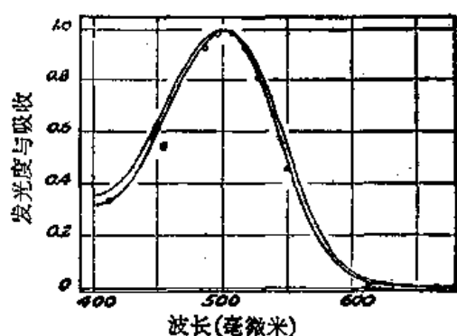
图 35-9 暗适应眼睛的灵敏度曲线和视锥的吸收曲线的比较
