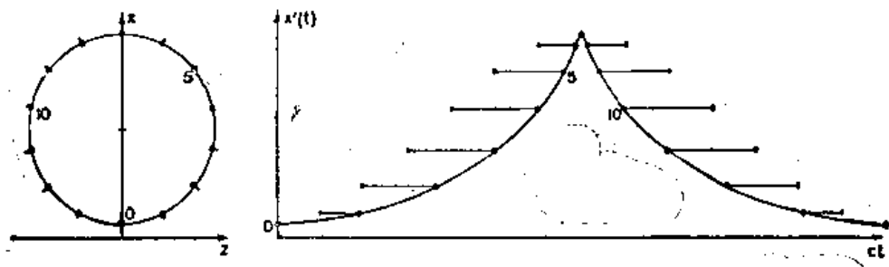
图 34-3 以恒定速率 v=0.94c 沿圆周运动的质点的 x'(t) 曲线
