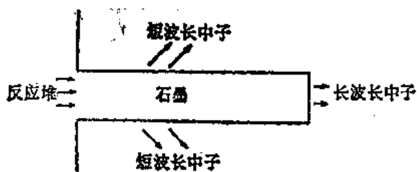
图 38-7 反应堆中子通过石墨块的扩散
