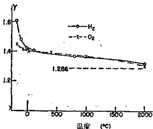
图 40-6 氢与氧的 \gamma 实验值与温度的关系。 经典理论预言 \gamma=1.286 ,与温度无关
