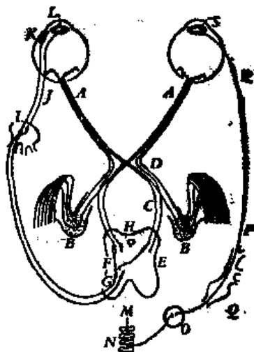
图 36-3 眼睛的机械动作的神经内部连结
