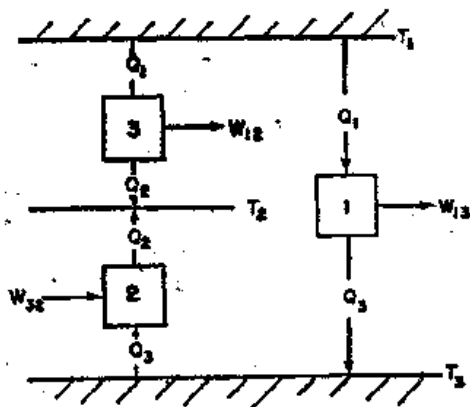
图 44-8 热机 1 与 2 联合起来等于热机 3
