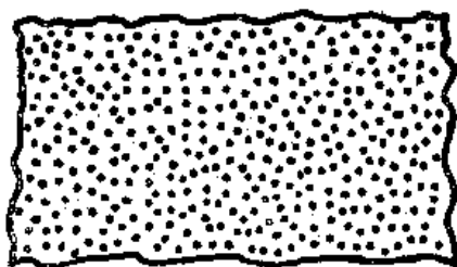
图 5-10 在只观察核的时候, 通过一块厚 1 厘米的碳所见到的那个设想的图象
