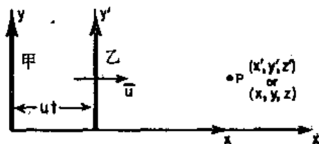
图 15-1 沿着 x 轴以均匀速度作相对运动的两个坐标系
