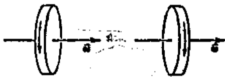
图 52-3 转轮与其镜像。注意角速度 “矢量”并没有反转
