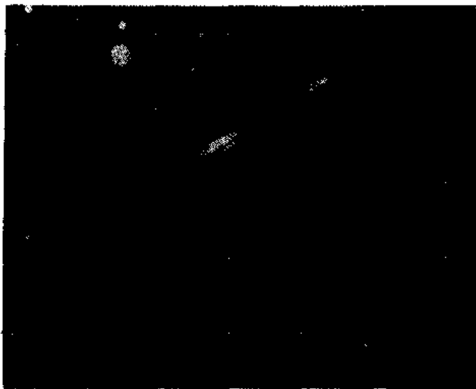
图 5-7 与我们的银河系一样的一个螺旋银河系，假定它的直径与我们的银河系相近，那么我们从它的表现大小就能算出它的距离。它离地球约 3000 万光年（即 3 \times 10^{23} 米）
