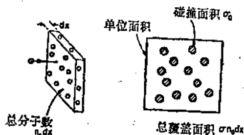
图 43-1 碰撞截面
