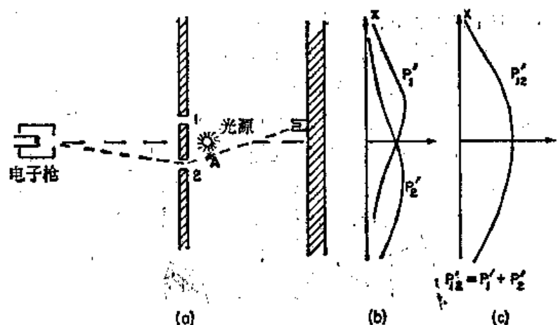
图 37-4 另一个电子的实验
