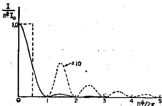
图 30-2 大量等幅度振子的总强度与相角的函数关系
