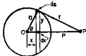
图 13-6 一个均匀带电的球壳的势能
