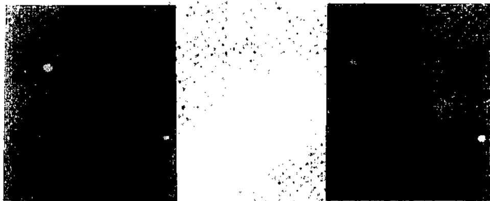
图 7-6 双星系统
