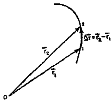
图 11-6 在短时间间隔 \Delta t = t_2 - t_1 内, 一个粒子的位移
