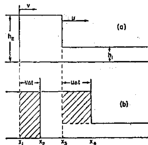
图 51-5 水槽中一个激浪的两个横截面, 其中(b)比(a)迟 \Delta t 时间
