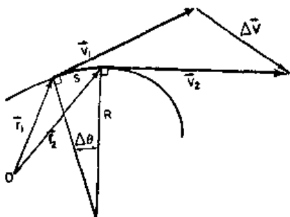
图 11-7 曲线轨道示意图
