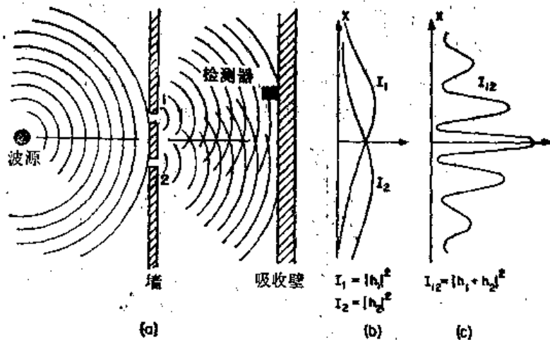
图 37-2 水波干涉实验
