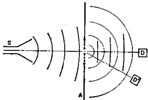
图 26-13 无线电波通过一个狭缝
