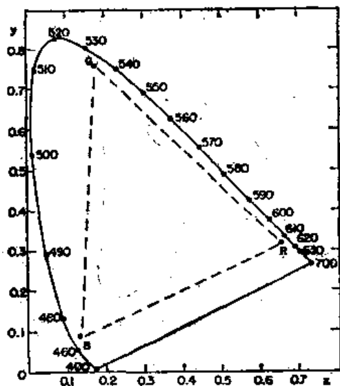
图 35-4 标准色品图
