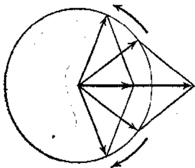
图 33-8 两个反向旋转的等幅矢量相加产生一方向固定但幅度振荡的矢量
