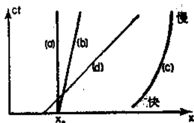
图 17-1 三个粒子在空-时中的轨迹:
