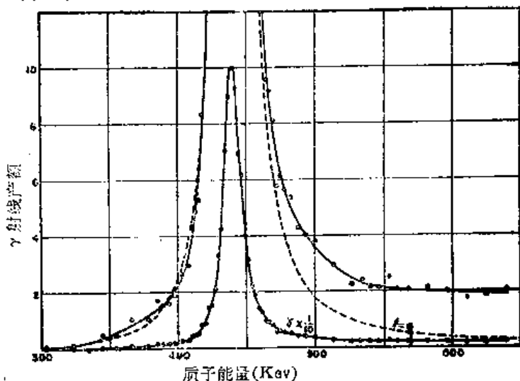
图 23-9 从锂原子中射出的 \gamma -射线强度与轰击质子能量的关系。 虚线是对角动量 l=0 的质子进行计算时得出的理论曲线
