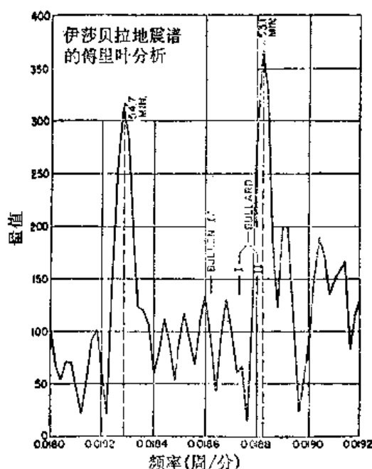
图 51-8 某一地震仪记录的高分辨率分析, 其中显示出双重谱线
