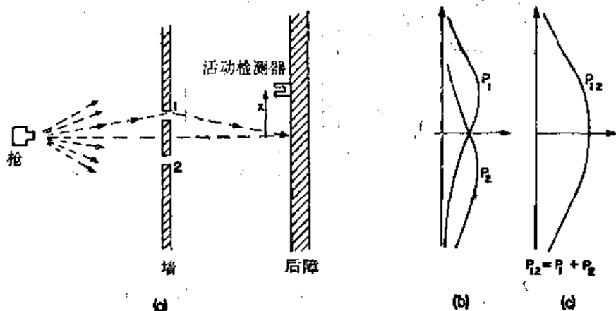
图 37-1 子弹的干涉实验
