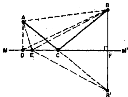
图 26-3 最短时间原理的说明
