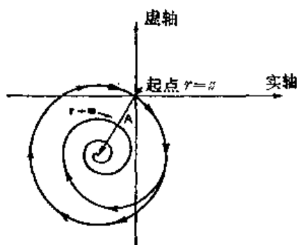
图 30-12 \int_z^\infty \eta e^{-i\omega r/c} dr 的图解
