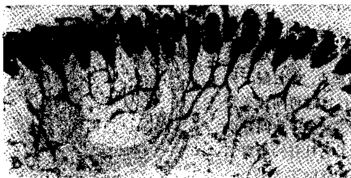
图 36-11 蜃的复眼。(a)上视图;(b)横截面
