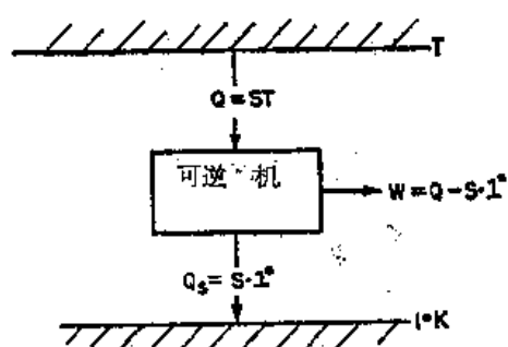
图 44-9 绝对热力学温度
