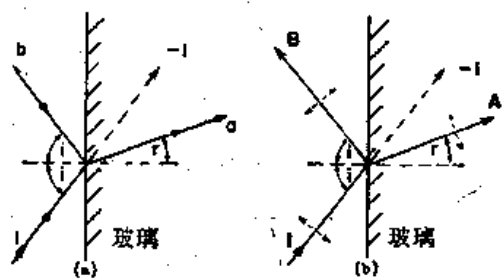
图 33-6 振幅为 1 的入射波在玻璃表面的反射与折射。(a) 中入射波垂直于纸面偏振。(b) 中入射波的线偏振方向用虚线电矢量表示
