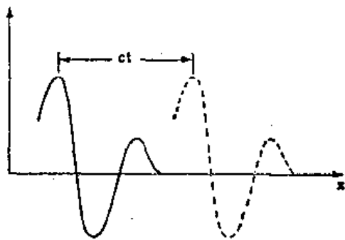
图 47-2 实线表示在某一瞬时电场的可能情况，虚线表示在时间 t 后的电场
