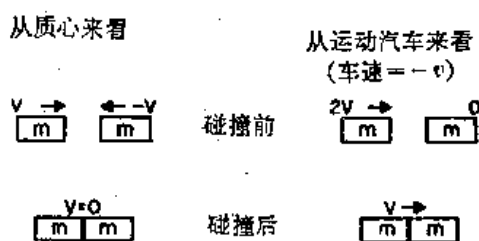
图 10-4 质量相等的物体进行的非弹性碰撞的两种情况
