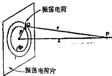
图 30-10 振荡电荷面的辐射场
