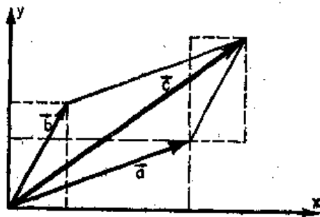
图 11-4 矢量加法
