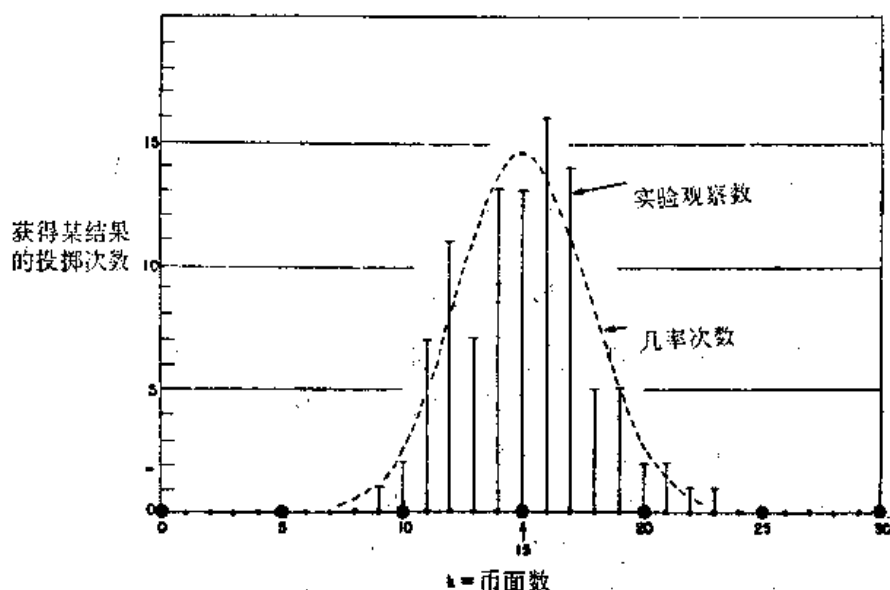
图 6-2 每轮 30 次抛掷的 100 轮游戏所得结果的概况。垂直线表示记录到 k 次正面的各轮游戏的数目。虚线表示从概率计算求得的所期望记录到 k 次的游戏轮数
