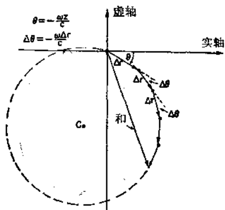
图 30-11 \int_0^\infty e^{-i\omega r/c} dr 的图解
