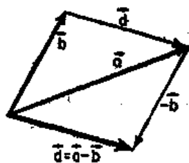
图 11-5 矢量的减法
