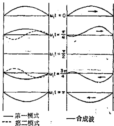
图 49-3 两种模式组合成一个行波
