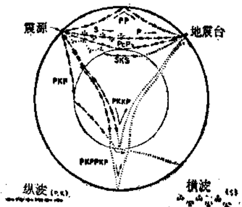
图 51-6 地球的示意图，表示纵声波和横声波的路径
