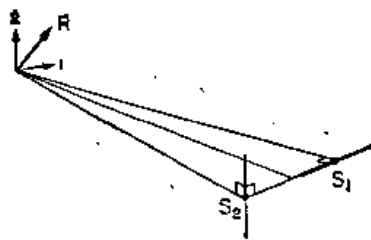
图 28-4 两个源迭加时的矢量特征示意图
