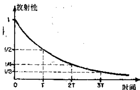
图5-3 放射性随时间而减小。在每一个“半衰期” T 中，放射性都减少一半
