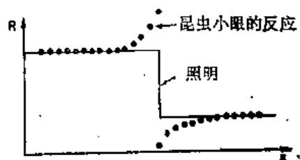
图 36-13 蜚的小眼在突然改变照明的地方附近的净反应
