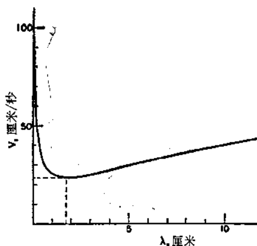
图 51-11 水波的相速度对波长的曲线
