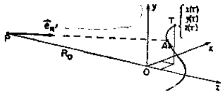
图 34-1 运动电荷的路径。在时刻 \tau 电荷的真正位置在 T ,但其推迟位置在 A
