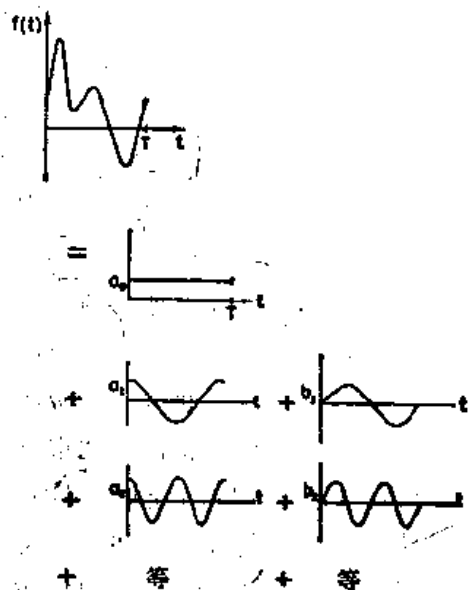
图 50-2 任何周期函数 f(t) 等于简谐函数之和
