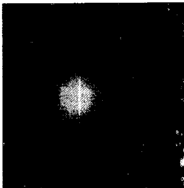
图 5-6 靠近我们银河系中心的一个星团。其中各恒星与地球的距离为 30,000 光年,或约为 3 \times 10^{21} 米
