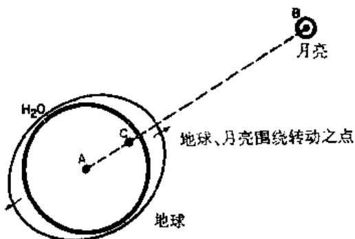
图 7-5 解释潮汐现象的地球——月球系统
