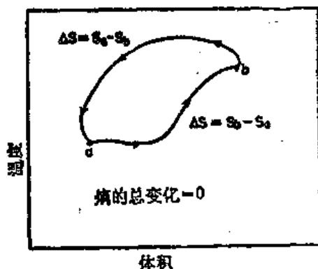
图 44-11 在完全可逆循环中熵的改变
