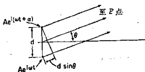
图 29-10 两个振幅相等、相互间有 \alpha 位相差的振子
