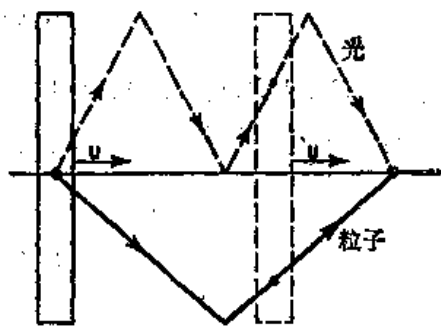
图 16-1 光和“粒子”在一只运动的钟内的运动轨迹
