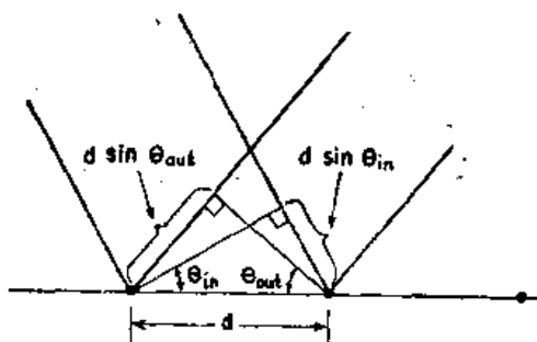
图 30-4 从光栅上相邻划线散射的光线的程差是 d \sin \theta_{out} - d \sin \theta_{in}
