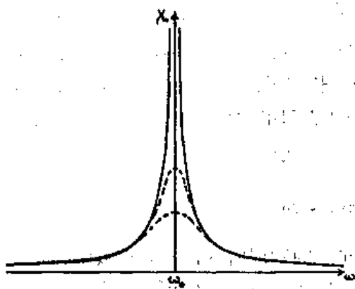
图 25-5 对应不同摩擦力的共振曲线
